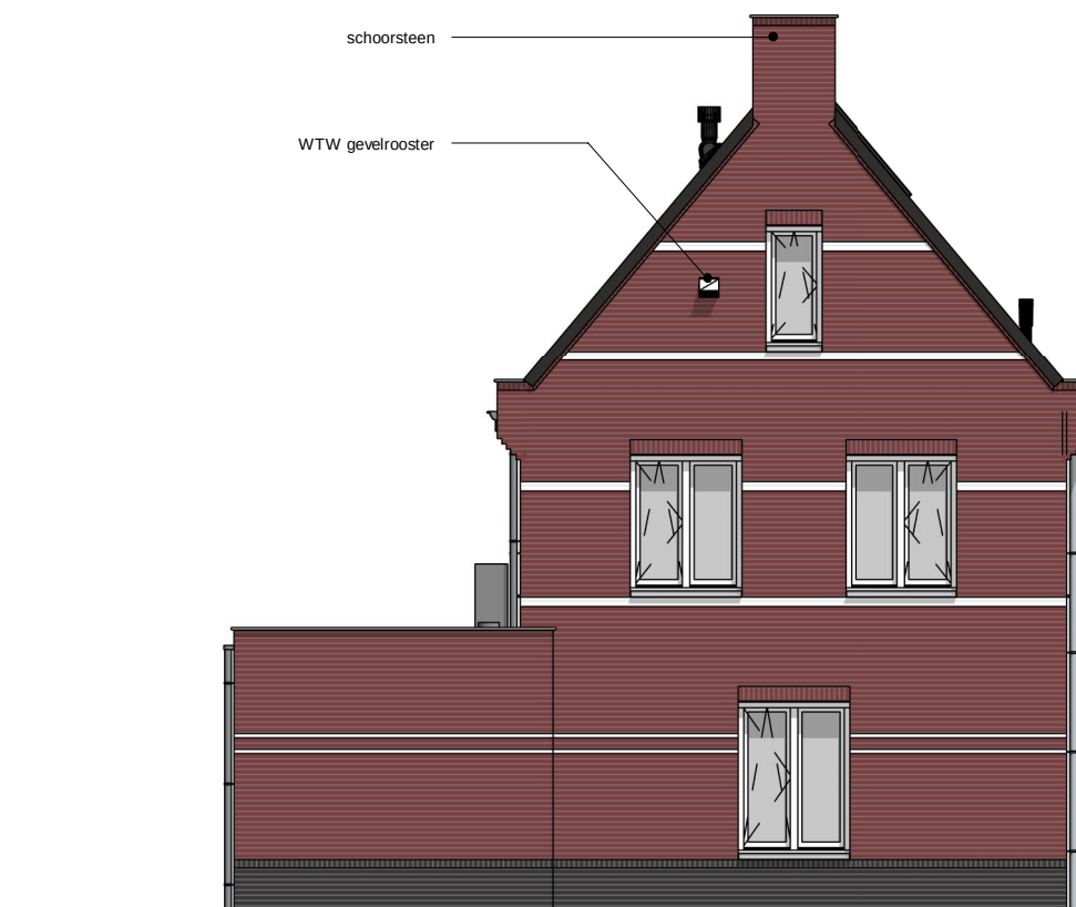
linkergevel schaal 1 : 100
