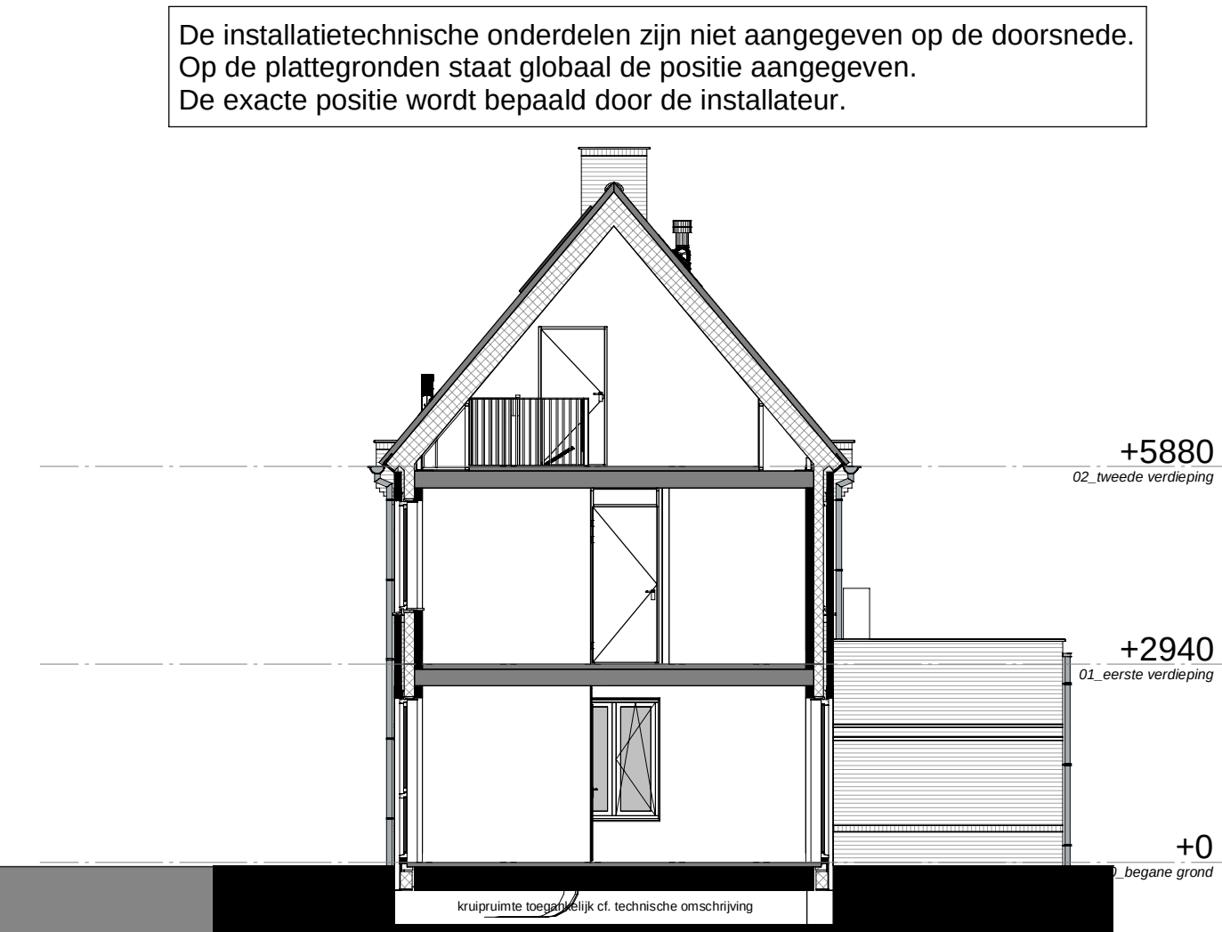
Doorsnede schaal 1 : 100
