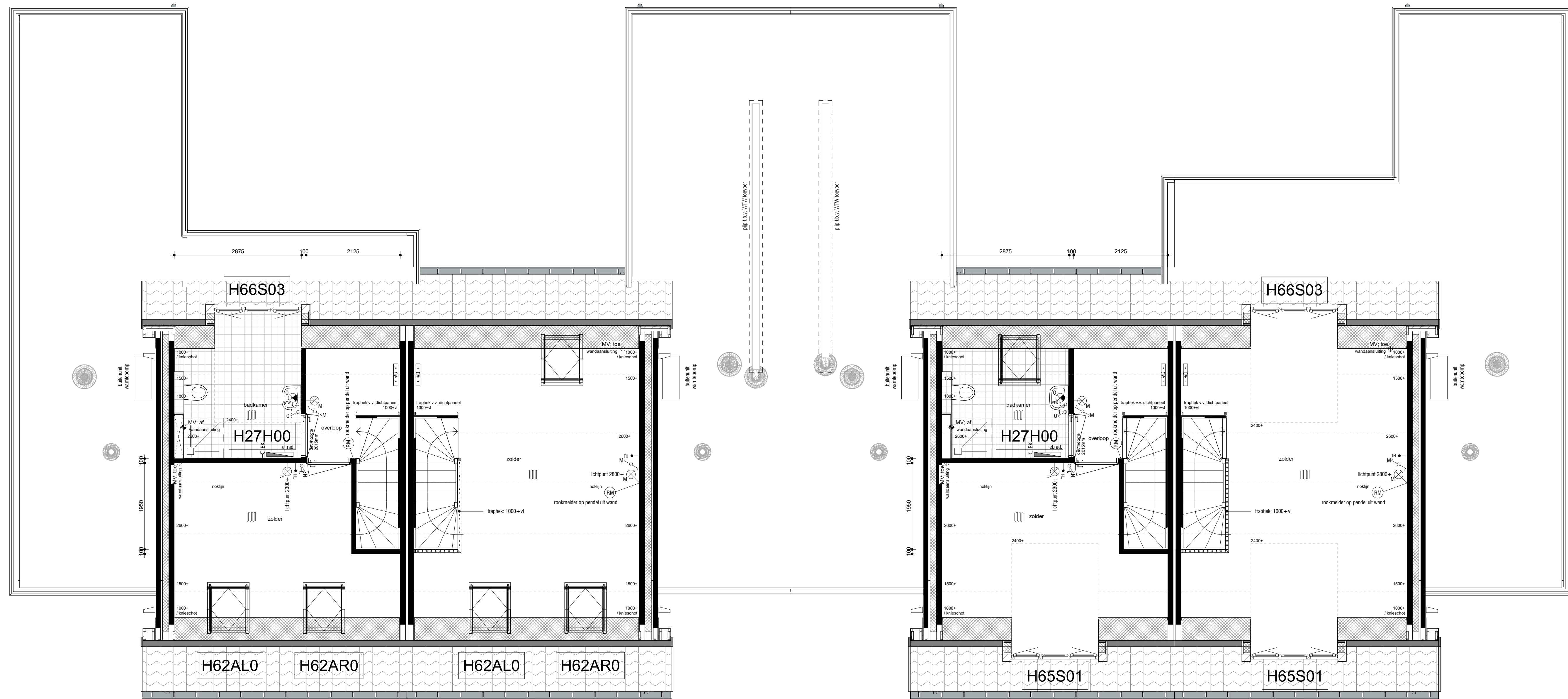
eerste verdieping schaal 1 : 50
