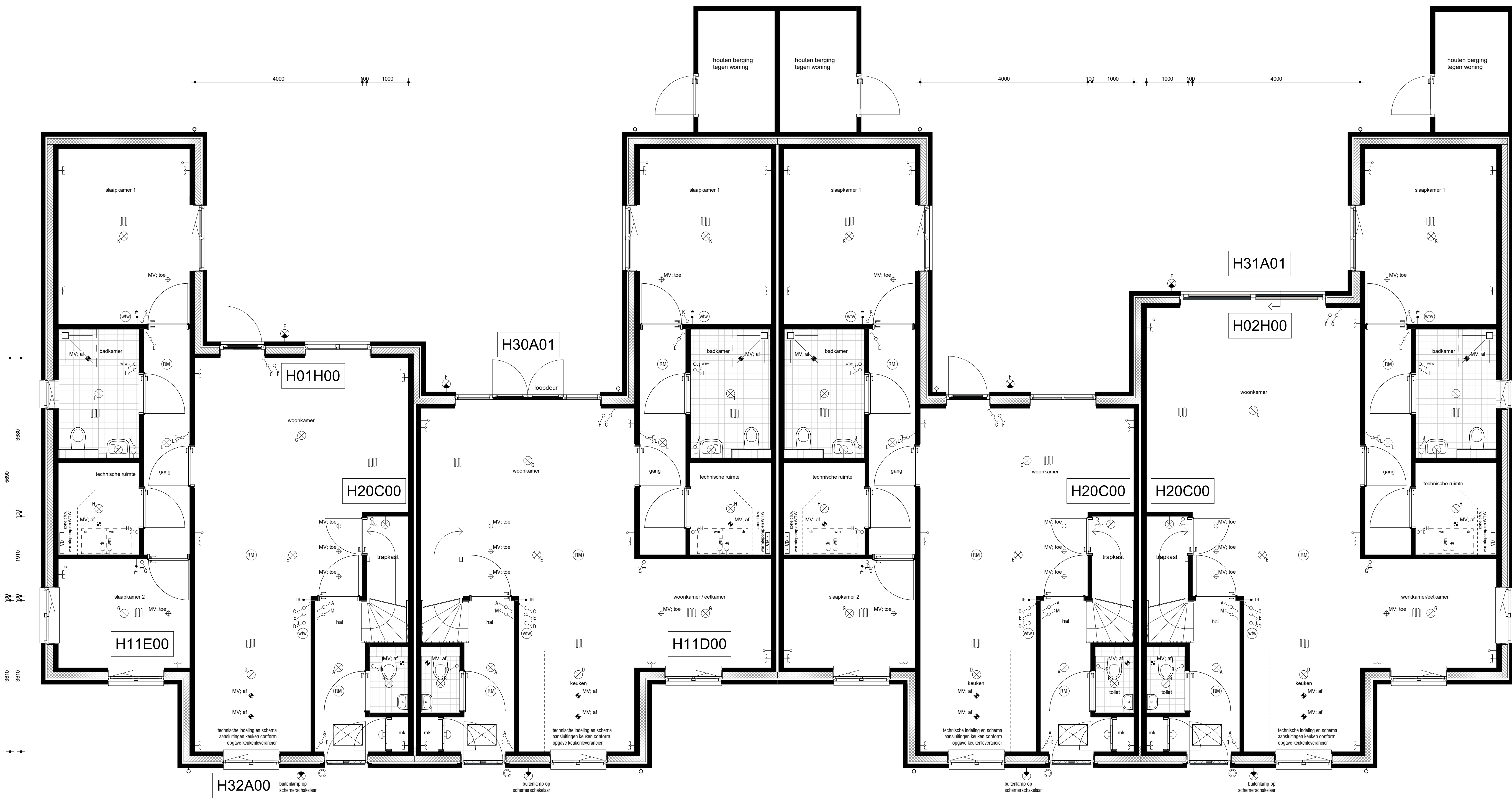
begane grond schaal 1 : 50
